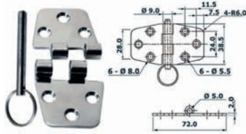
Scharnier type 4 met uitneembare pin
